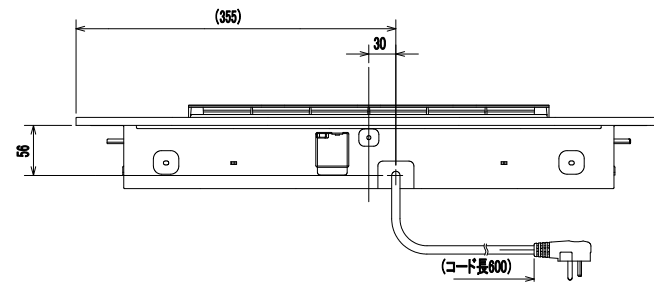
【背面図】
