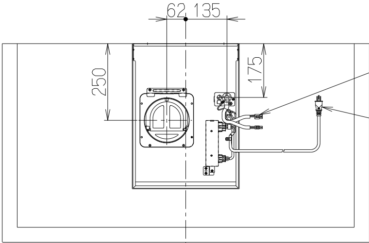
スイッチ部拡大図 (S=1/3)
