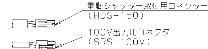
連動線詳細図
