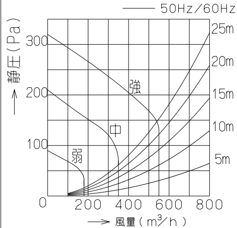
静圧-風量 曲線
